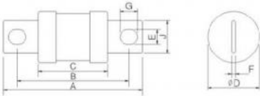
CFG1 500V DC 35A-800A
