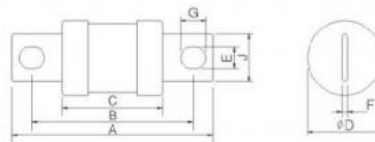
CFG1 500V DC 35A-800A
