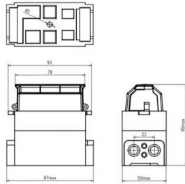
HRC100 II a/II b SP (适配 II a、II b熔断体) (For II a、II b fuselink) 图1 Fig. 1
